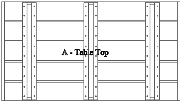
( 1 ) - One Table Top STSA-EPT4-A-01
